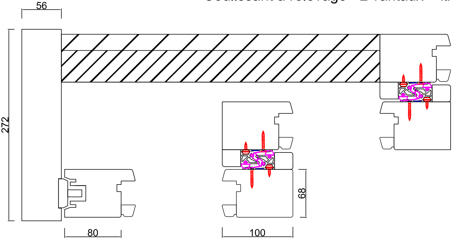
Coulissant à relevage - 2 vantaux + fixe
