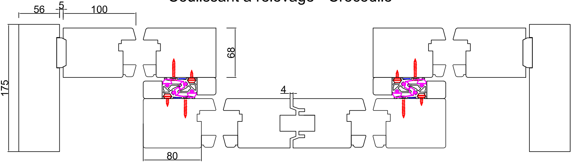
Coulissant à relevage - Crocodile
