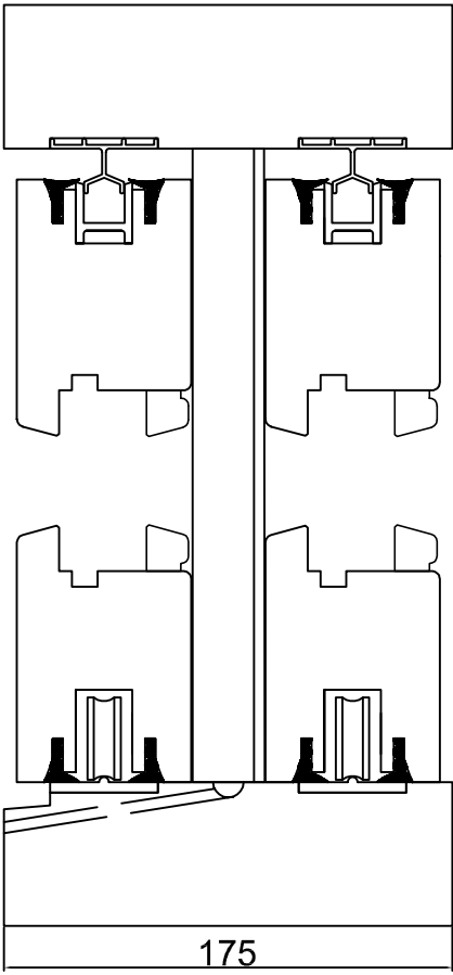
Seuil Bois
