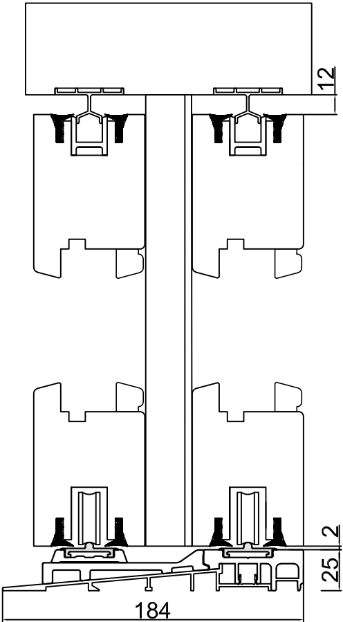
Seuil ALU
